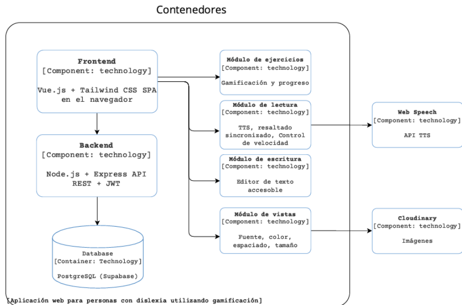
Ilustración 29. Diagrama de contenedores.
